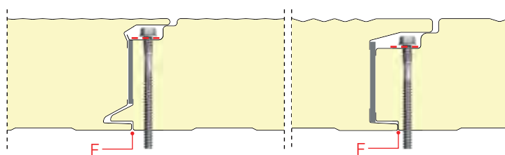
Dettaglio del giunto
