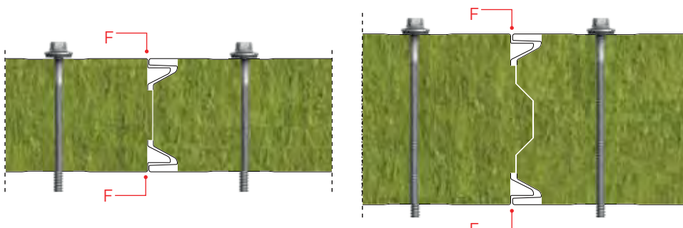
Dettaglio del giunto
