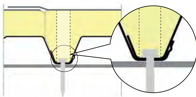
Dettagli del sistema di fissaggio
