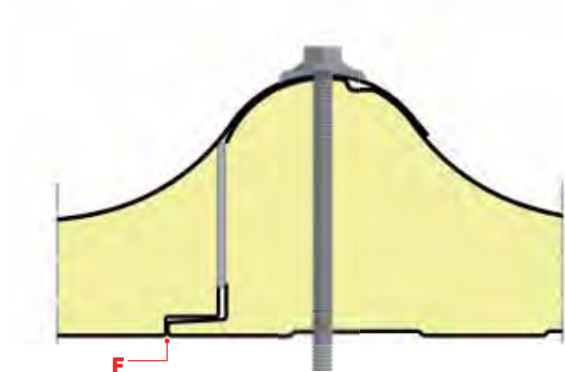
Dettaglio del sistema di accoppiamento e incastro
